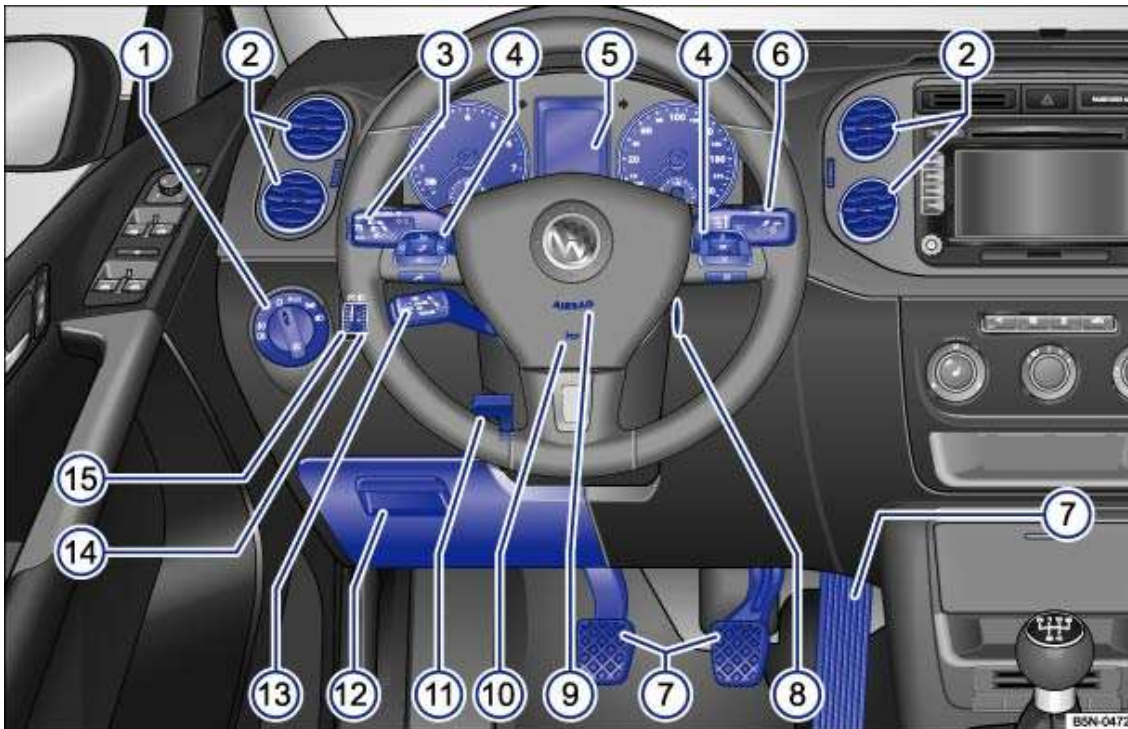
Abb. 5 Übersicht der Fahrerseite (Linkslenker).
