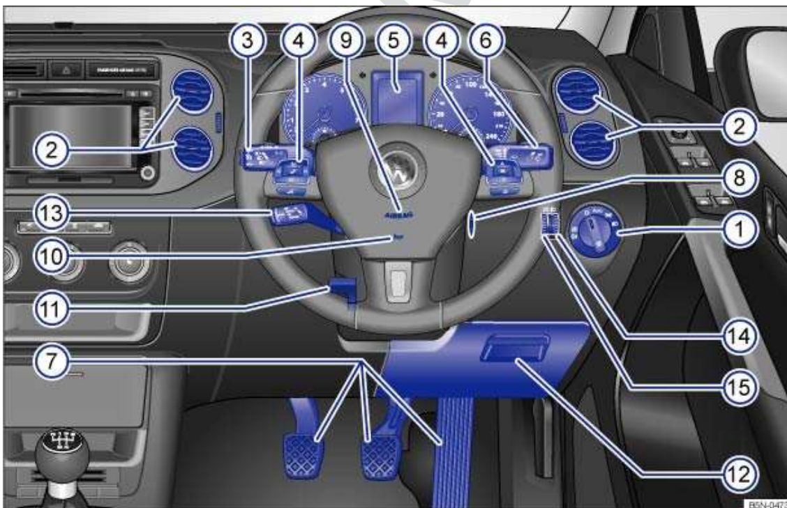
Abb. 6 Übersicht der Fahrerseite (Rechtslenker).
